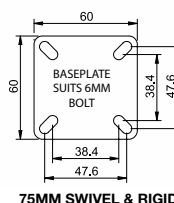
75MM SWIVEL & RIGID
